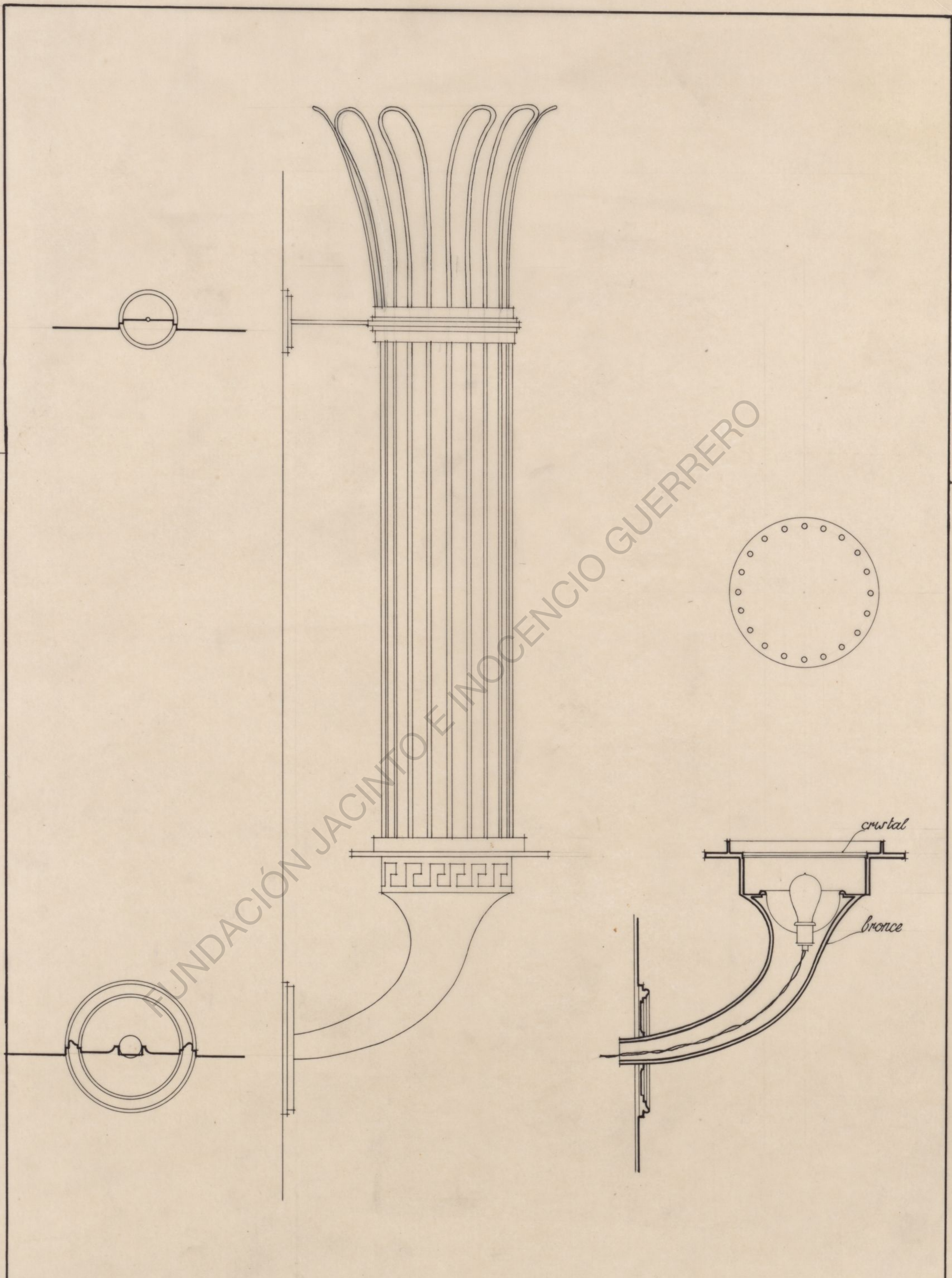
FAROL DE ENTRADA EN EL VESTIBULO DEL TEATRO COLISEUM MADRID ESCALA 1:10
